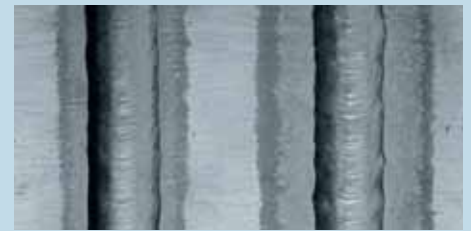
Lichtbogenstabilisierung durch VARIGON® S (links) im Vergleich zu Argon (rechts)
