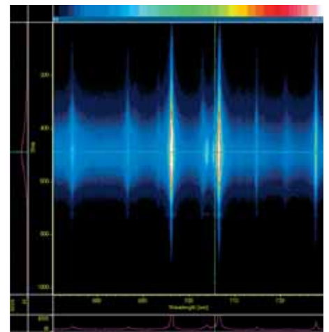
Einsatz wissenschaftlicher Forschungsmethoden zur Untersuchung plasmaphysikalischer Vorgänge im Lichtbogen: Ausschnitt einer Spektralanalyse am MIG-Schweißprozess von Aluminium mit VARIGON® He30S
