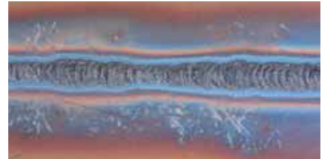
WIG-Naht, Wurzelseite unformiert
